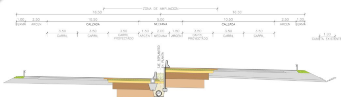
SECCIÓN TIPO TRONCO PRINCIPAL "A-49"
