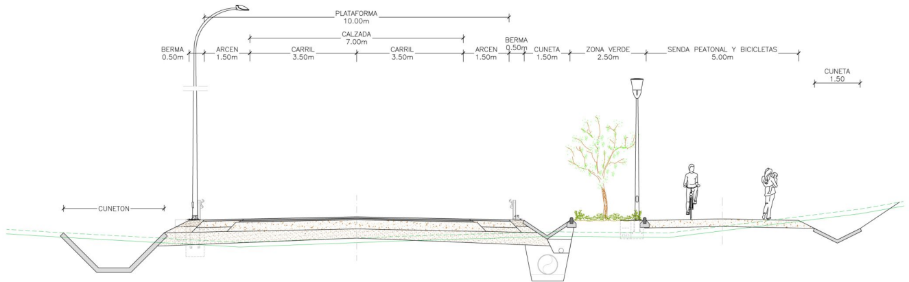
SECCION TIPO TRAMO 2
